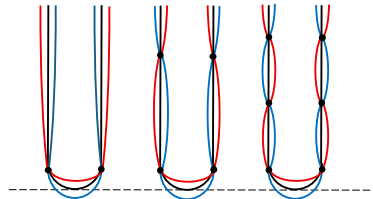
Rysunek 22. Schematyczne drgania ramion kamertonu dla kilku pierwszych drgań nieharmonicznych Źródło: opracowanie własne.
