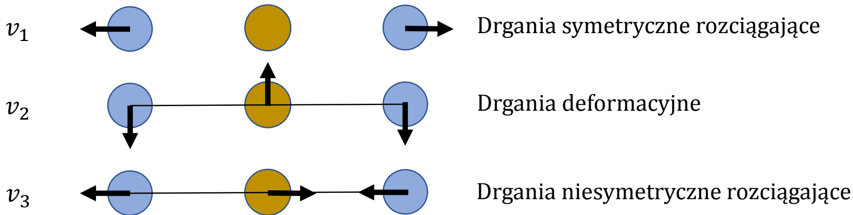
Rys. 4.3. Trzy podstawowe typy drgań cząsteczki CO 2 [1,2].
