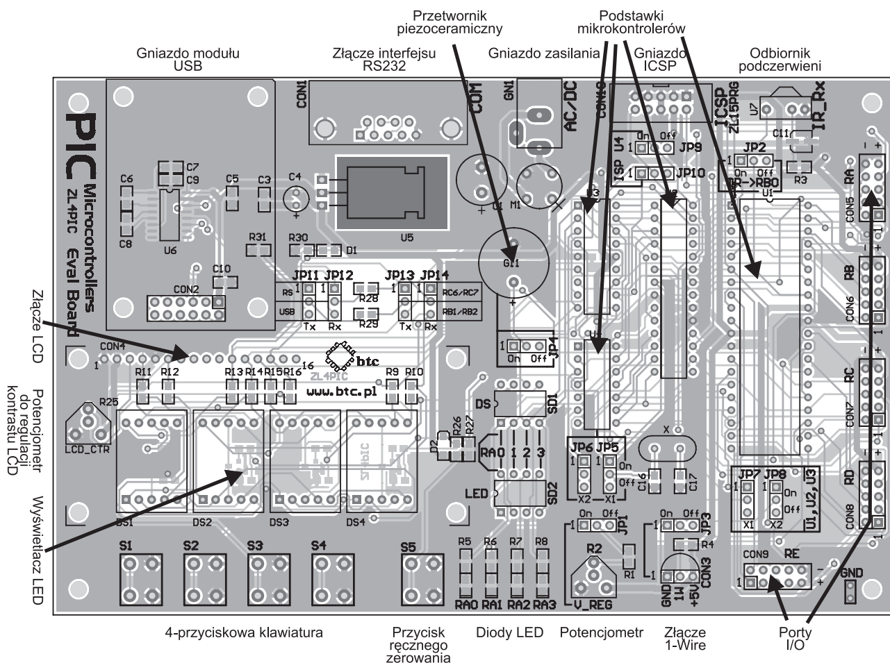
Rys. 3. Rozmieszczenie najważniejszych elementów zestawu
