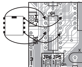
Rys. 2. Sposób montowania mikrokontrolerów w obudowach DIP8 w podstawce U4
