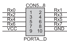
Rys. 4. Rozmieszczenie wyprowadzeń portów PORTA...D na złączach IDC
